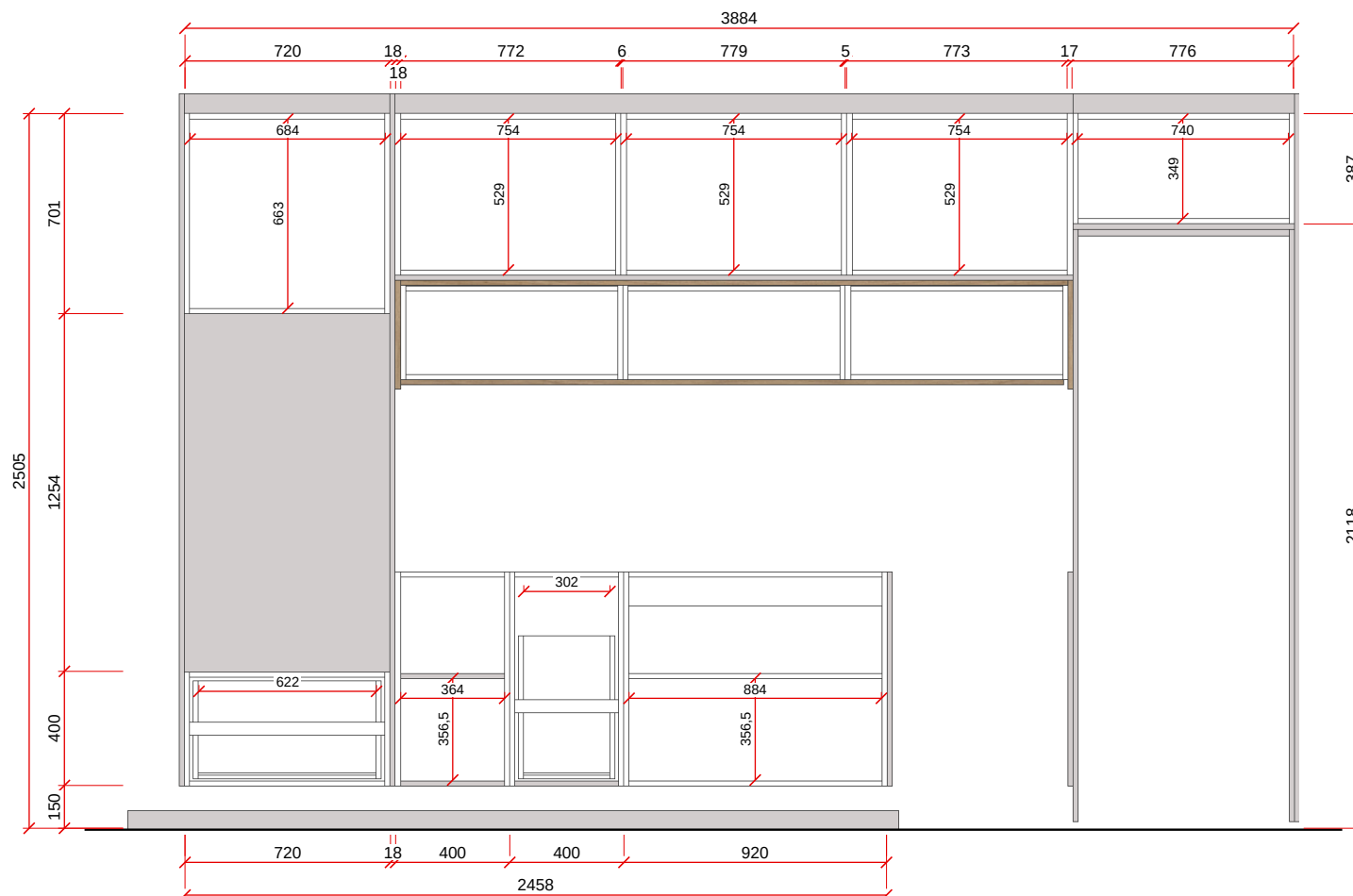
VISTA B - ESC. 1:25
